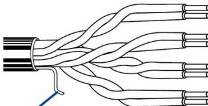
С рипкордом 4-парный кабель
